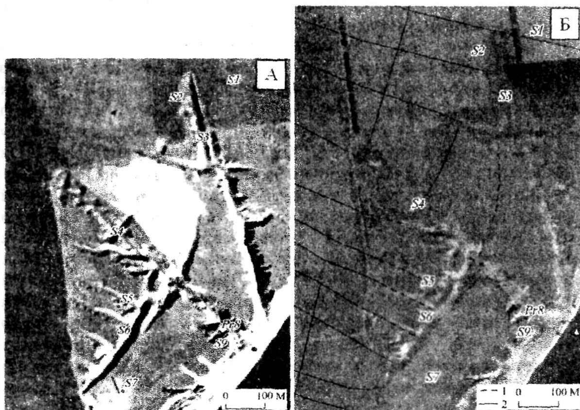
Рис. Сопряженность следов античного размежевания земель с антропогенно обусловленными эрозионными формами (А) и реконструкция античного землеустройства (Б) в урочище “Крестовый овраг”.
