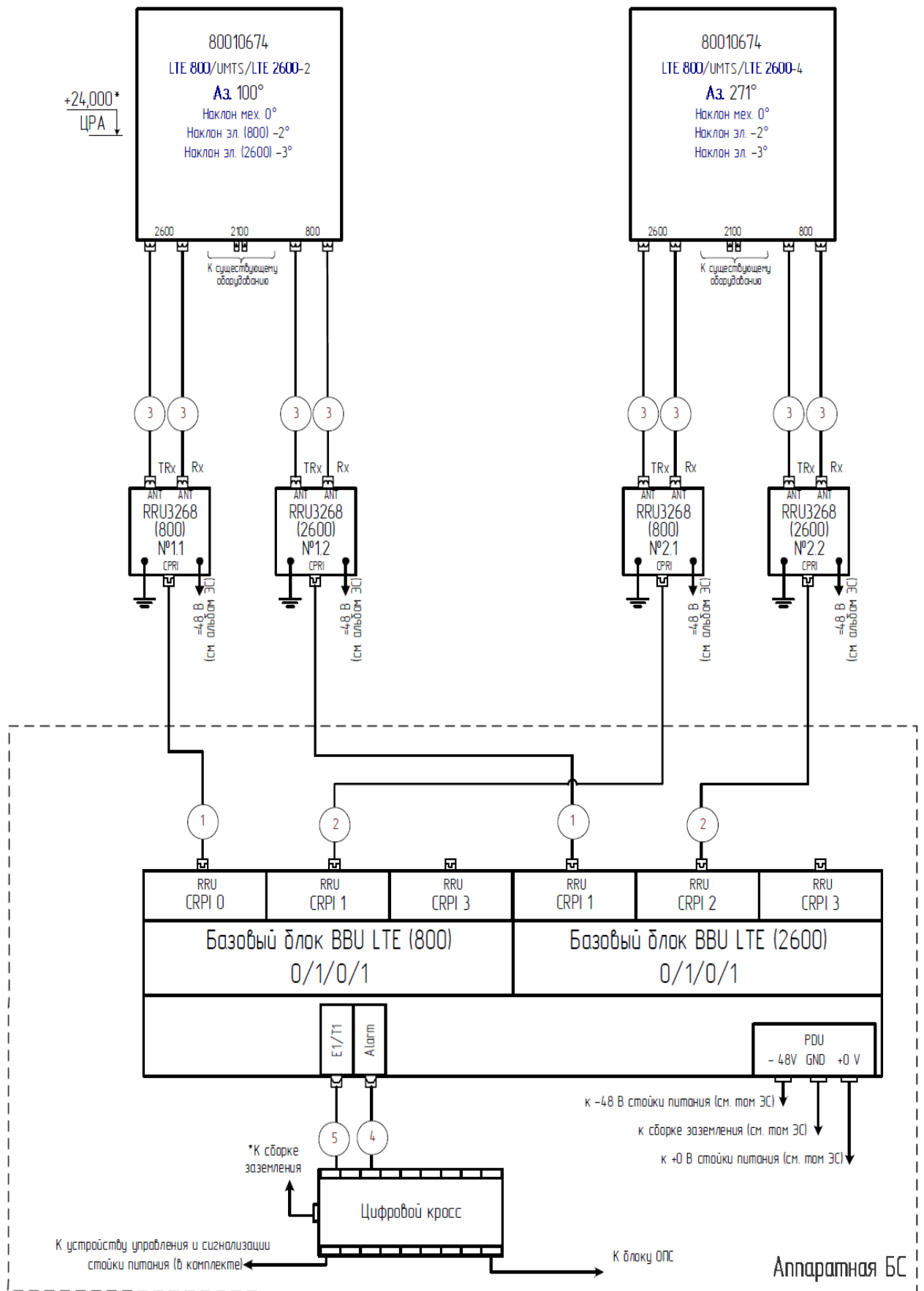
Рисунок 3.3 – Схема подключения базовой станции
