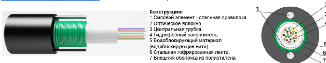
Рисунок 3.7 – Оптический кабель ОККЦ(н)
