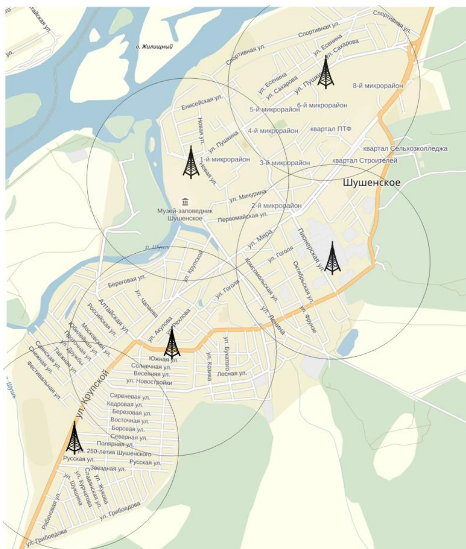
Рисунок 3.6 – Планируемое размещение базовых станций в пгт.Шушенское
