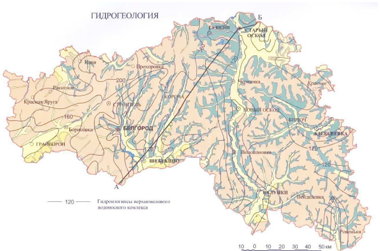
Рисунок 1.3.1- Гидрогеологическая карта Белгородской области.
