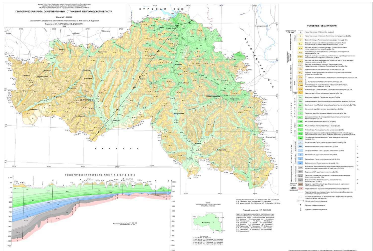
Рисунок 1.2-Геологическая карта дочетвертичных отложений Белгородской области.
