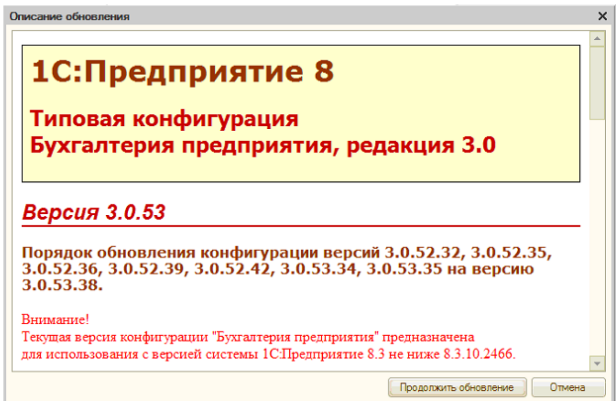
Рисунок 5 – описание обновления
