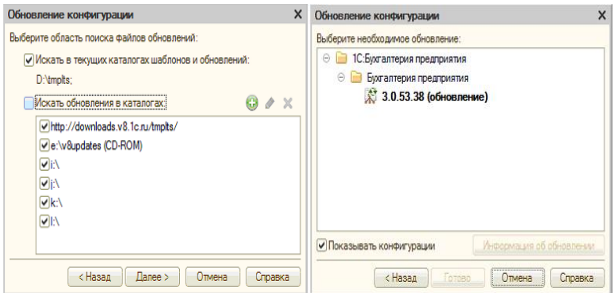
Рисунок 4 – выбор обновления
