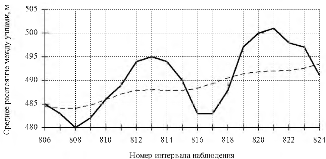
Рис. 2. Результаты аппроксимации с помощью авторегрессионной модели Fig. 2. Approximation results using an autoregressive model
