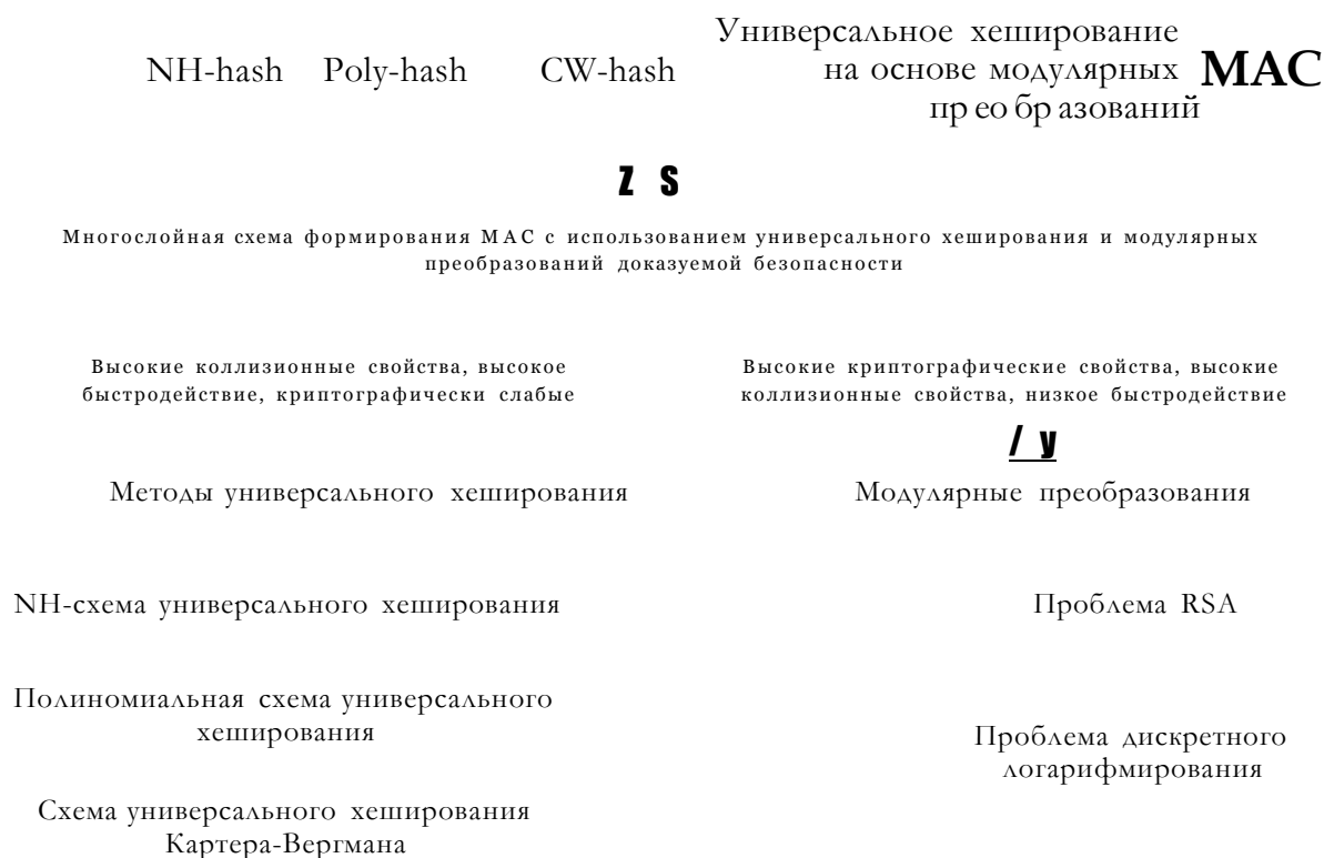
Рис. 3. Предлагаемая схема каскадного формирования кодов контроля целостности и аутентичности данных с использованием модулярных преобразований
