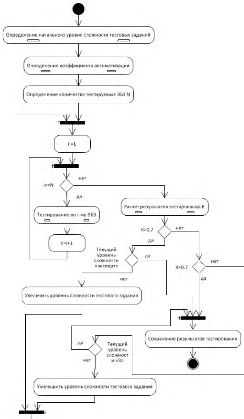
Рис. 2. Алгоритм адаптивного тестирования
