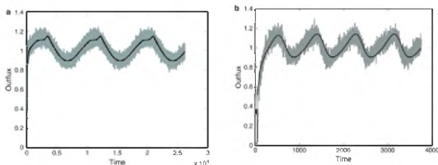
Рис. 6. Сравнение решений PDE-модели и DES-модели, Lefebvre E. 2010 Fig. 6. Comparison of PDE-model and DES-model, Lefebvre E. 2010
