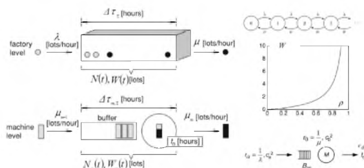
Рис. 2. Основные параметры TQ-модели [19, p.10] Fig. 2. The basic parameters TQ-model [19, p.10]
