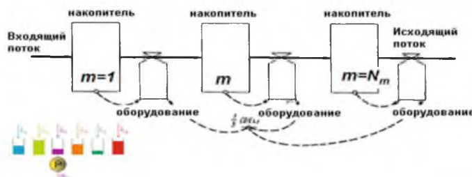
Рис. 3. Концептуальное представление Fluid-модели [6] Fig. 3. Conceptual view of Fluid-model [6]
