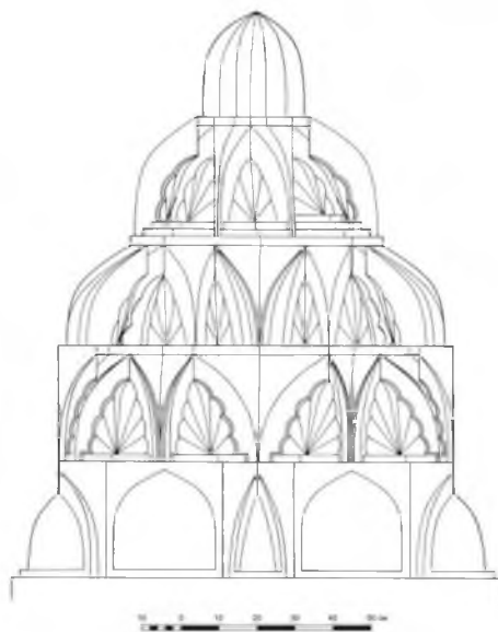
Рис. 3. Конха михраба. Вид спереди. Реконструкция. Рисунок авторов Fig. 3. Concha of Mihrab. Front view. Reconstruction. Drawing of the authors
