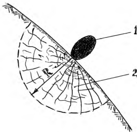
Рис. 2. Схема к расчету температурного режима при аккреции: 1 – планетезималь; 2 – зона деформирования формирующейся Земли
