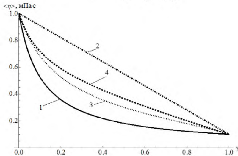
Рис. 1. Вилка Фойгта-Рейсса [\langle \eta \rangle_F, \langle \eta \rangle_R] и Кравчука-Тарасюка [\underline{\langle \eta \rangle}, \overline{\langle \eta \rangle}] оценки разброса вязкости двухкомпонентной смеси несжимаемых жидкостей ( \eta_1 = 0.1 \text{ мПа} \cdot \text{с} , \eta_2 = 0.1 \text{ мПа} \cdot \text{с} ) в зависимости от концентраций компонент \gamma :
