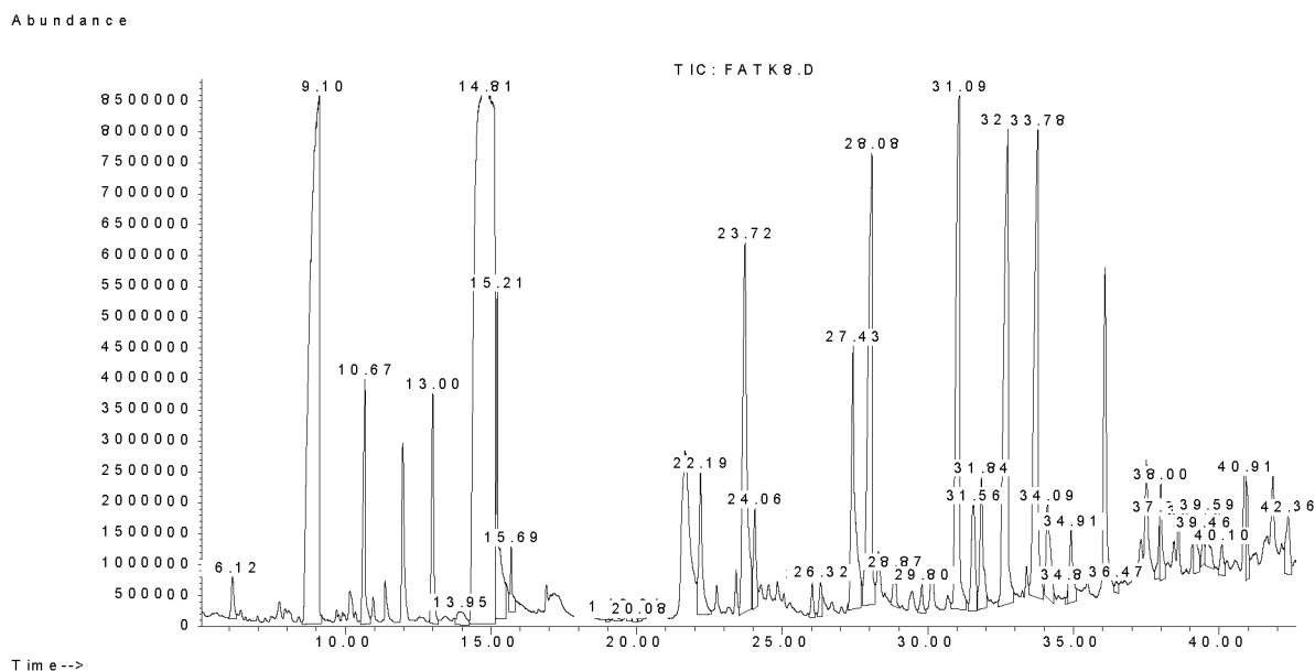
Рис. 1. Схема хроматограммы газо–жидкостной– хромато–масс–спектрометрии жирных кислот травы колокольчика круглолистного Fig. 1. Schematic diagram of the chromatogram-mass spectral analysis of Fatty Acids of the herb of Bellflower ( Campanula rotundifolia L.)
