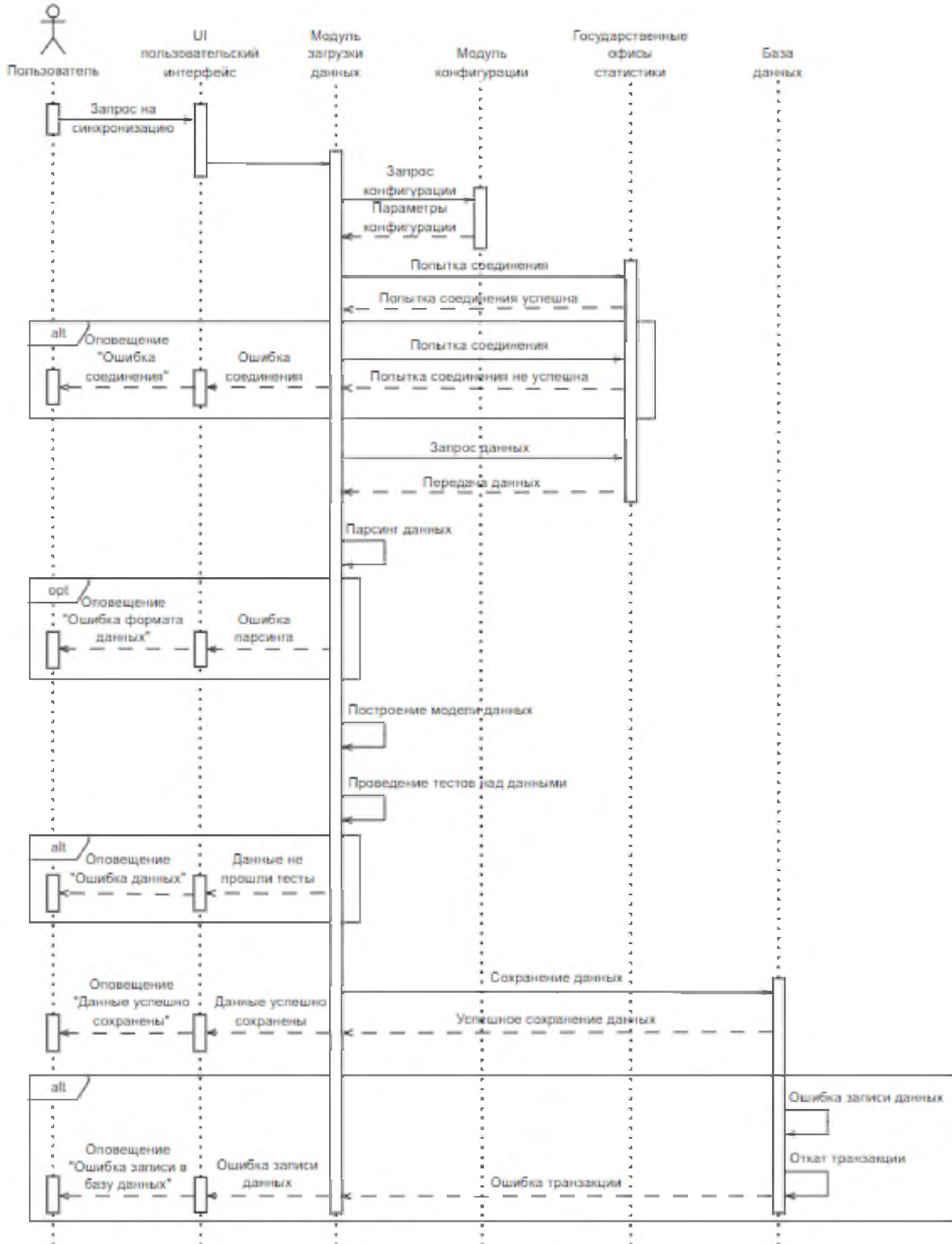
Рис. 3. UML-диаграмма последовательности работы модуля загрузки данных Fig. 3. UML diagram of the sequence of the data loading module operations
