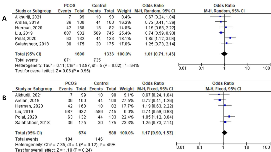
Рис. 5. Форест-график: ассоциация полиморфизма rs4880 с риском СПКЯ для рецессивной модели (СС против ТС + ТТ). А, В: с исследованием Liu и без него, соответственно
