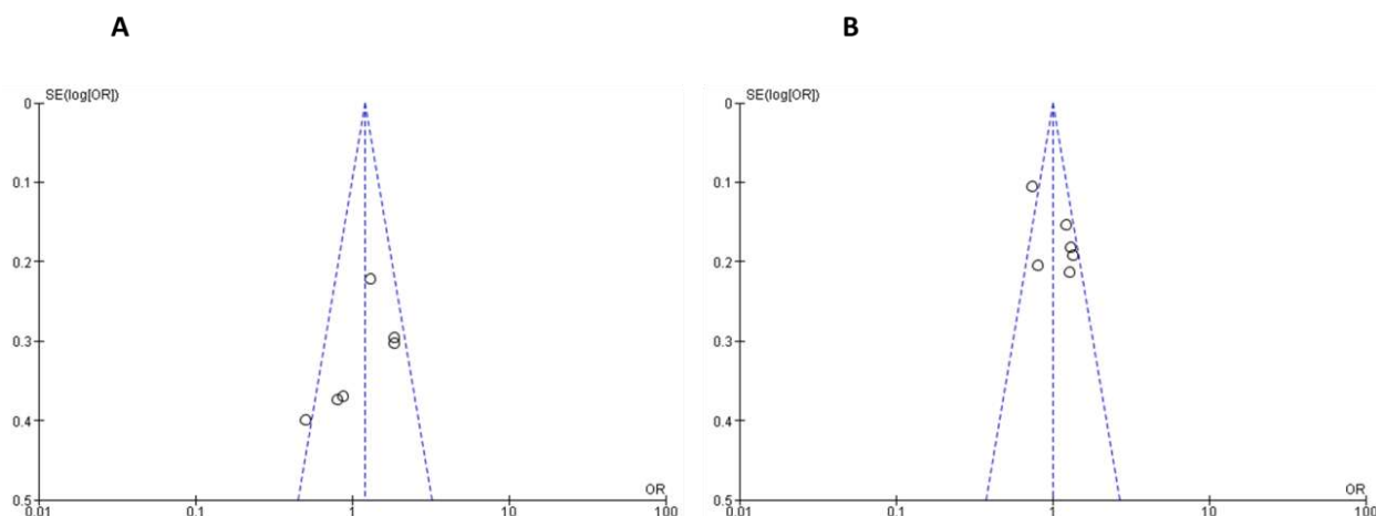
Рис. 7. Схема воронкообразных графиков для поиска ошибки публикации.
