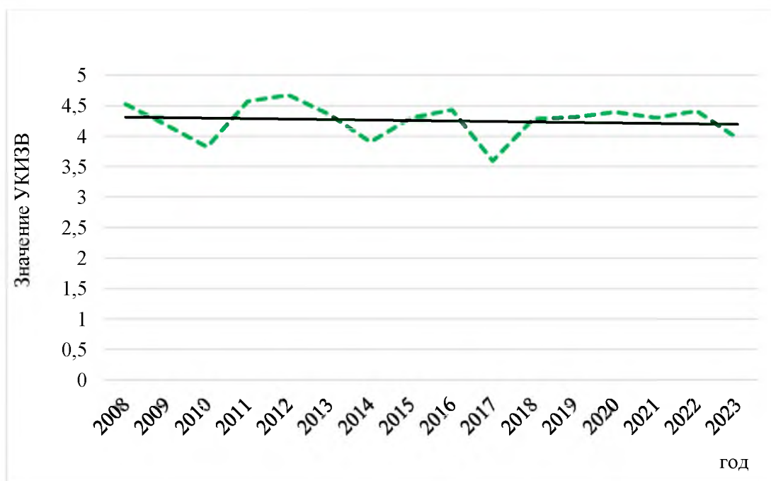
Рис. 2. Динамика удельного комплексного индекса загрязнённости воды в р. Везёлка
