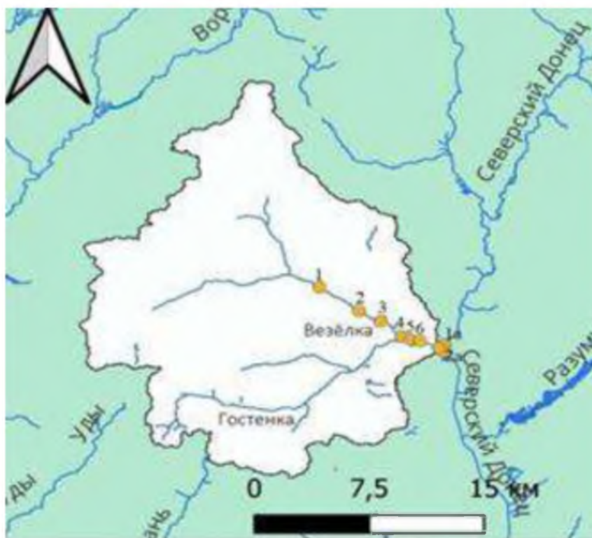
Рис. 1. Река Везёлка со створами наблюдения (№№ 1–6) и р. Северский Донец (№№ 1а–2а)
