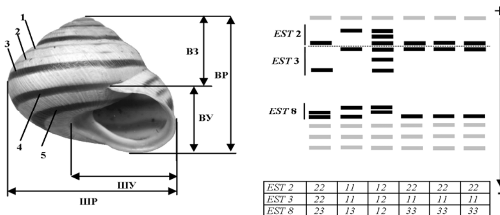
Рис. 2. Слева – раковина C. vindobonensis (промеры: ВР – высота раковины; ШР – ширина раковины; ВЗ – высота завитка; ВУ – высота устья; ШУ – ширина устья, 1–5 номера полос). Справа – зоны активности трех локусов эстераз и соответствующие им генотипы C. vindobonensis (серыми полосами обозначены мономорфные фракции)
